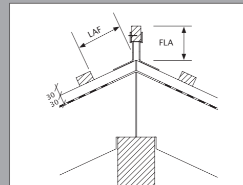
LAF = Lattenabstand zum Firstschnittpunkt (in mm) FLA = Firstlattenabstand (in mm)
