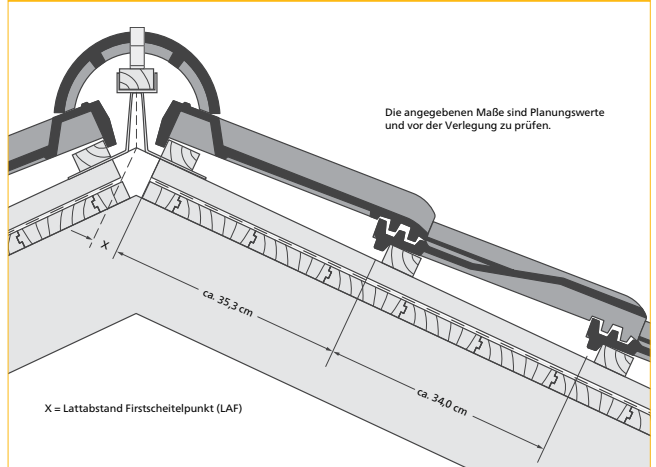
Firstziegel Nr. 15 mit Firstanschlussziegeln und Flächenlüfterziegeln
